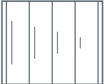
SIGNATURE 4 lignes progressives 1000 / 750 / 500 / 250 x 13 de hauteur (en mm)
