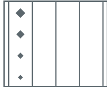
EVOLUTION 4 carrés progressifs 180 x 180 / 140 x 140 / 100 x 100 / 60 x 60 (en mm)
